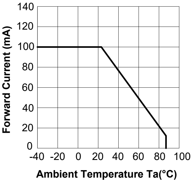
图.1 正向电路与环境温度
