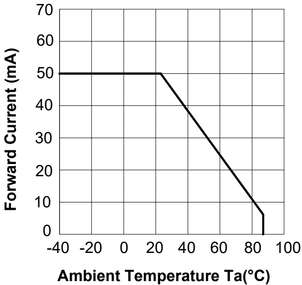
图.1 正向电路与环境温度
