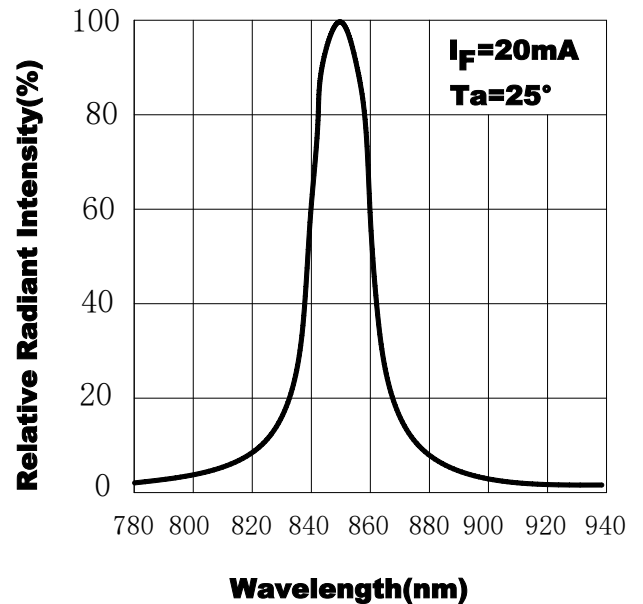
图.2 频谱分布
