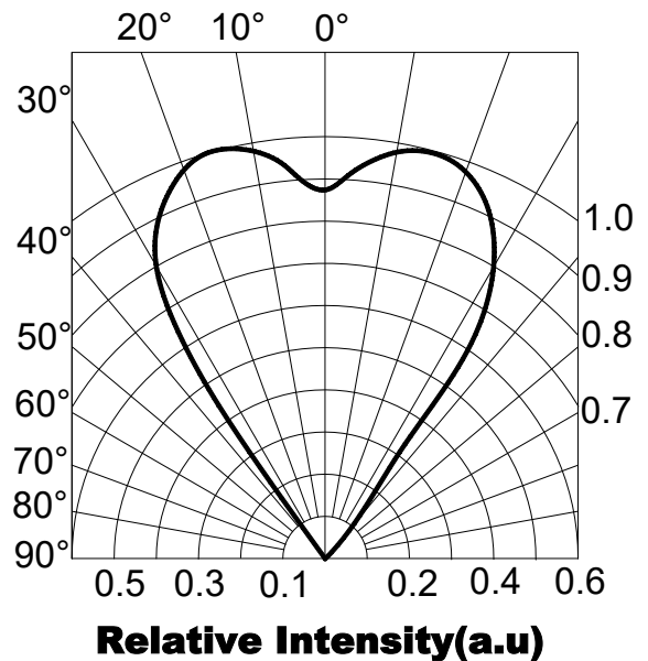
图.6 相对辐射强度与发射角度
